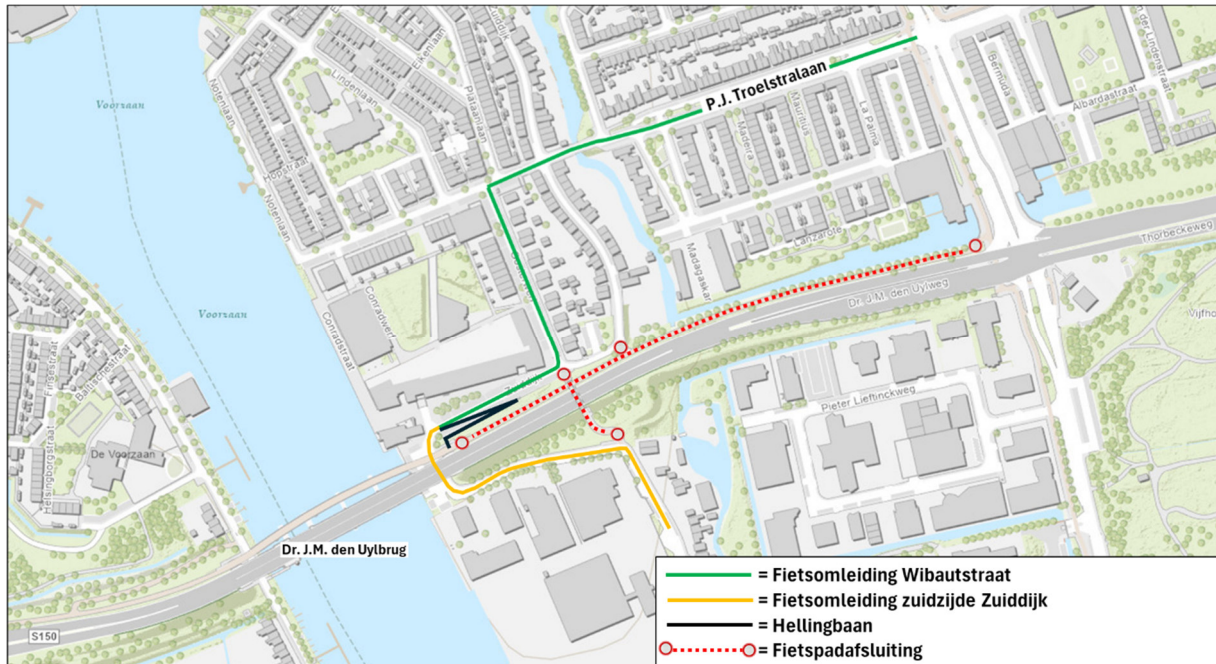
Afbeelding 3: Omleiding fietsers
